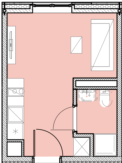
Rzut apartamentu Jednostki Typu A2
